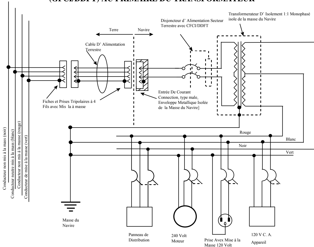
FIGURE 11-2 CIRCUIT D'UN TRANSFORMATEUR D'ISOLEMENT AVEC ENTRÉE MONOPHASE 240 VOLTS ET SORTIE MONOPHASÉE 120/240 VOLTS AVEC LA PROTECTION D' UN DISJONCTEUR DIFFERENTIAL (GFCI/DDFT) AU PRIMAIRE DU TRANSFORMATEUR
