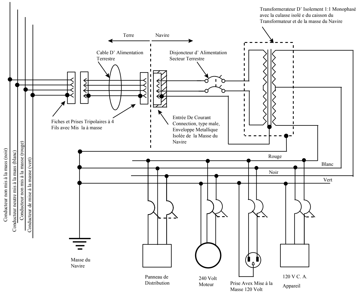
FIGURE 11-1 CURCUIT D'UN TRANSFORMATEUR D'ISOLEMENT AVEC ENTRÉE MONOPHASE 240 VOLTS ET SORTIE MONOPHASÉE 120/240 VOLTS
