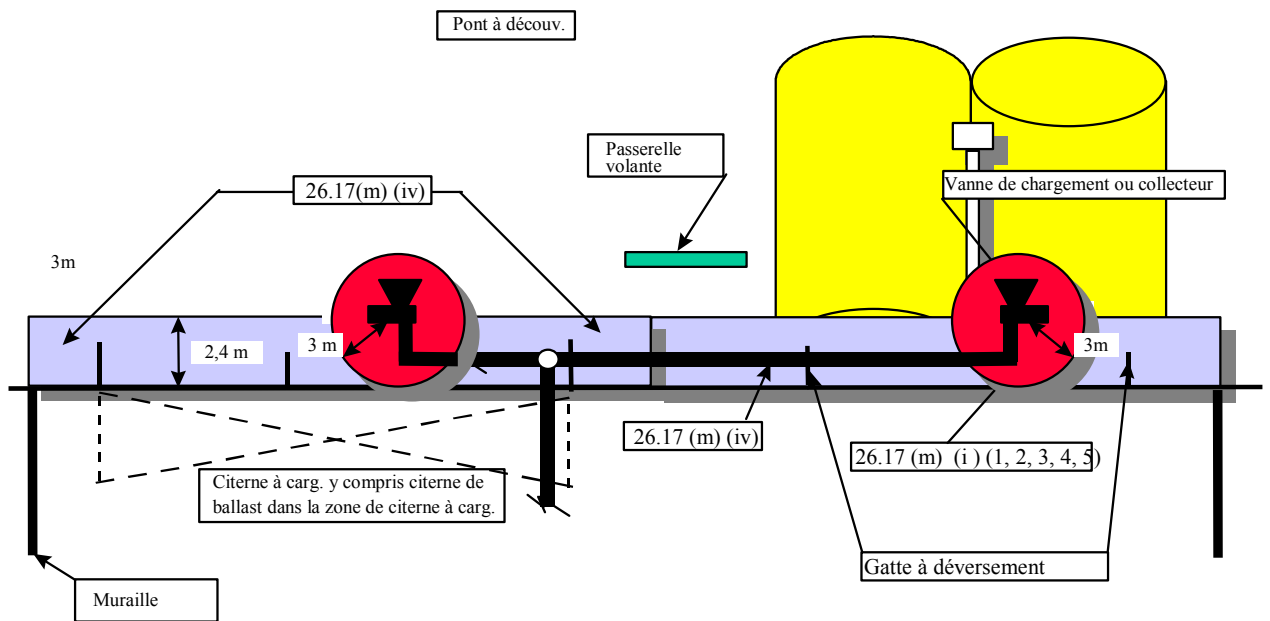
Vue en coupe de la citerne à cargaison et du pont à découvert
